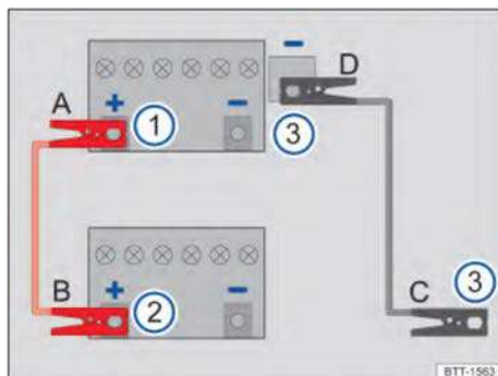
تصویر ۱۷۱ تصویر اتصال کابل‌های باتری به باتری
